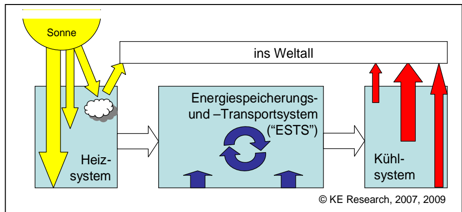
Abb 14: Der Energiehaushalt der Erde (schematisches Rollenmodell). Das Heizsystem regelt die Energiezufuhr von der Sonne zum Erdboden. Das Kühlsystem bewirkt die Abstrahlung ins Weltall. Alle „internen“ Transportvorgänge von Energie betrachten wir als Teil des „ESTS“.
